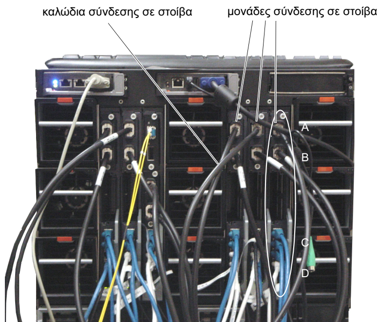
Εικόνα 1-1. Σύνδεση μεταγωγέων σε συνδεσμολογία στοίβας
